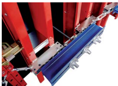
Detalle de paso de varilla diwidag. Este paso de varilla se hace por la viga de soporte, consiguiendo así darle rigidez al sistema.
